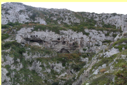
Fig. 90. Unita' costiera 106 (Canale del Ciolo).
